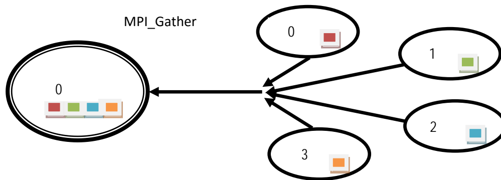
Figura 2.3. Esquema de trabajo de la función MPI_Gather .
