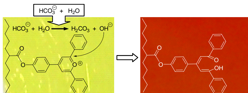
Figura 18. Representación del mecanismo sensor propuesto (filme 1). Se muestran los colores reales del polímero 1 en ausencia y en presencia del anión hidrogenocarbonato.
