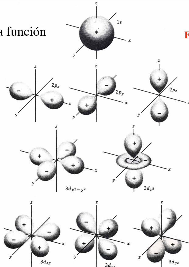
Figura 2-15 Representaciones tridimensionales que muestran la dependencia angular de los orbitales 1s , 2p y 3d para n fijo. [F. Daniels and R. A. Alberty, Physical Chemistry , 4.ª ed., pág. 416, John Wiley et Sons, Inc., New York (1975).]
