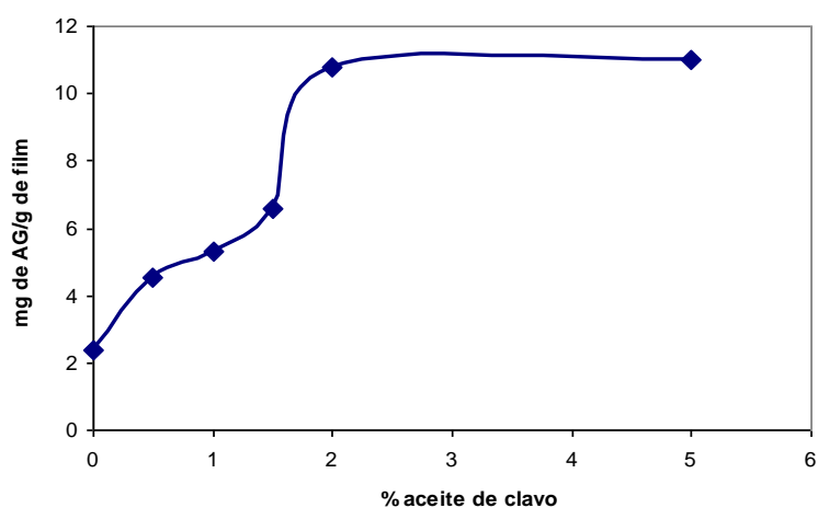
Figura 4: Concentración de polifenoles totales (expresados en mg de ácido gálico (AG)/g de film) de films de quitosano con diferentes concentraciones de aceite de clavo.
