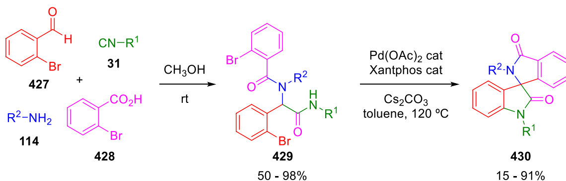
Scheme 86 Van der Eycken synthesis of spiranes
